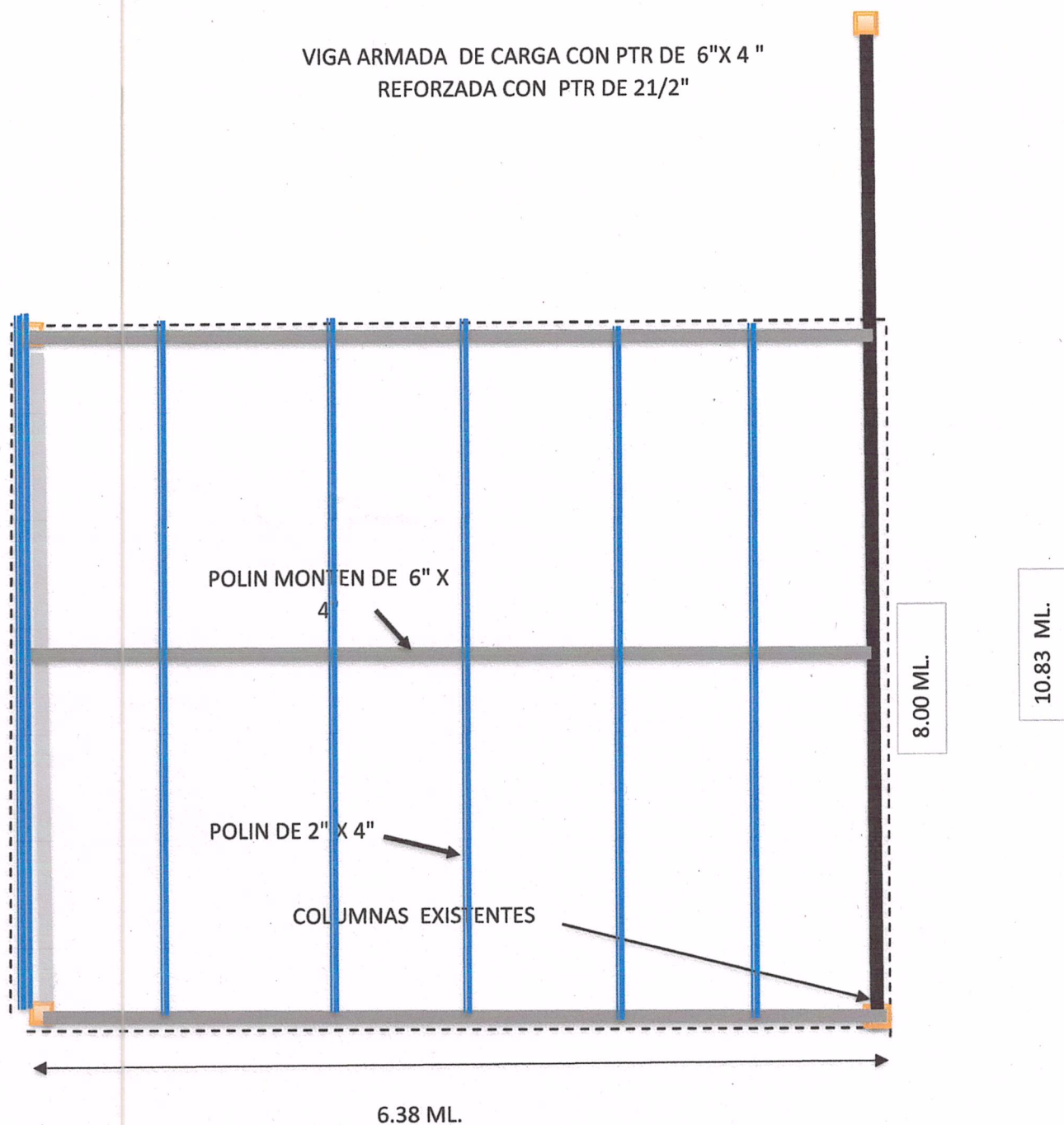
PLANTA ARQUITECTONICA
