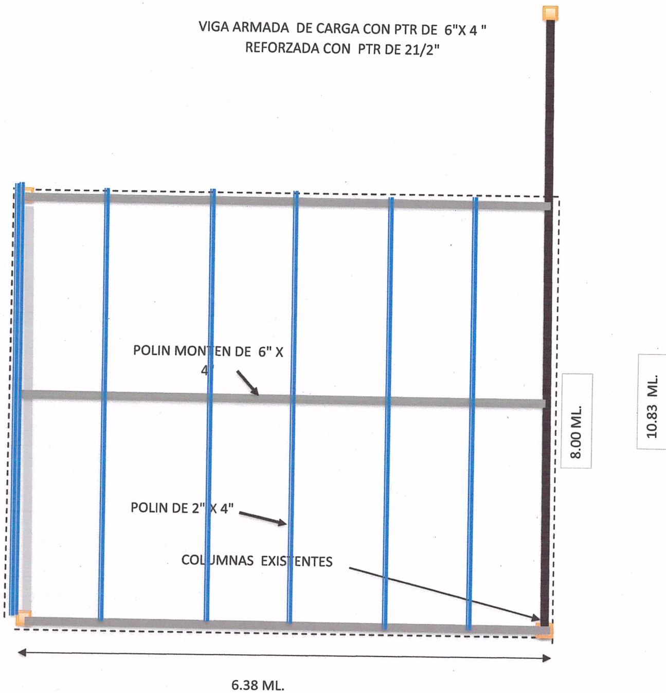
PLANTA ARQUITECTONICA
